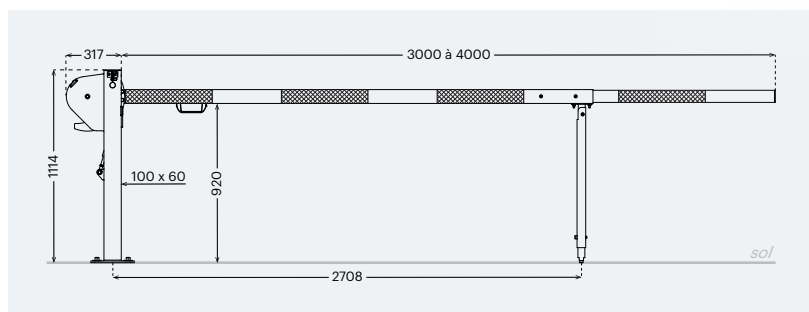
La traverse coulisse pour adapter la barrière au lieu de pose
